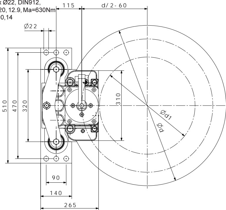
Schnitt A-A
